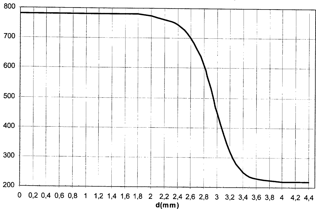
HV0,3 Filiation sur la zone 1 du moyeu C70 après trempe superficielle
